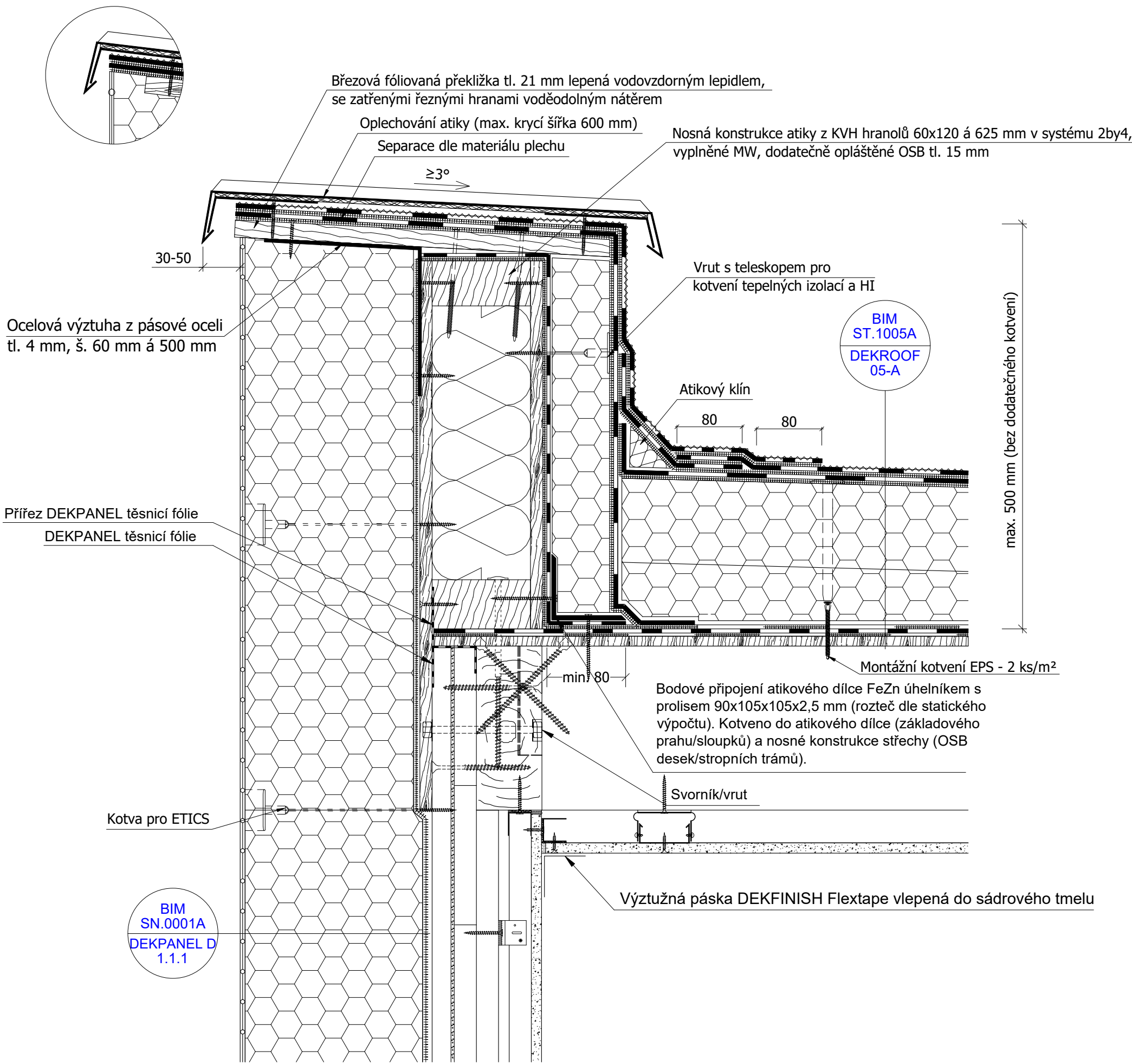
Alternativní řešení ukončení ETICS
