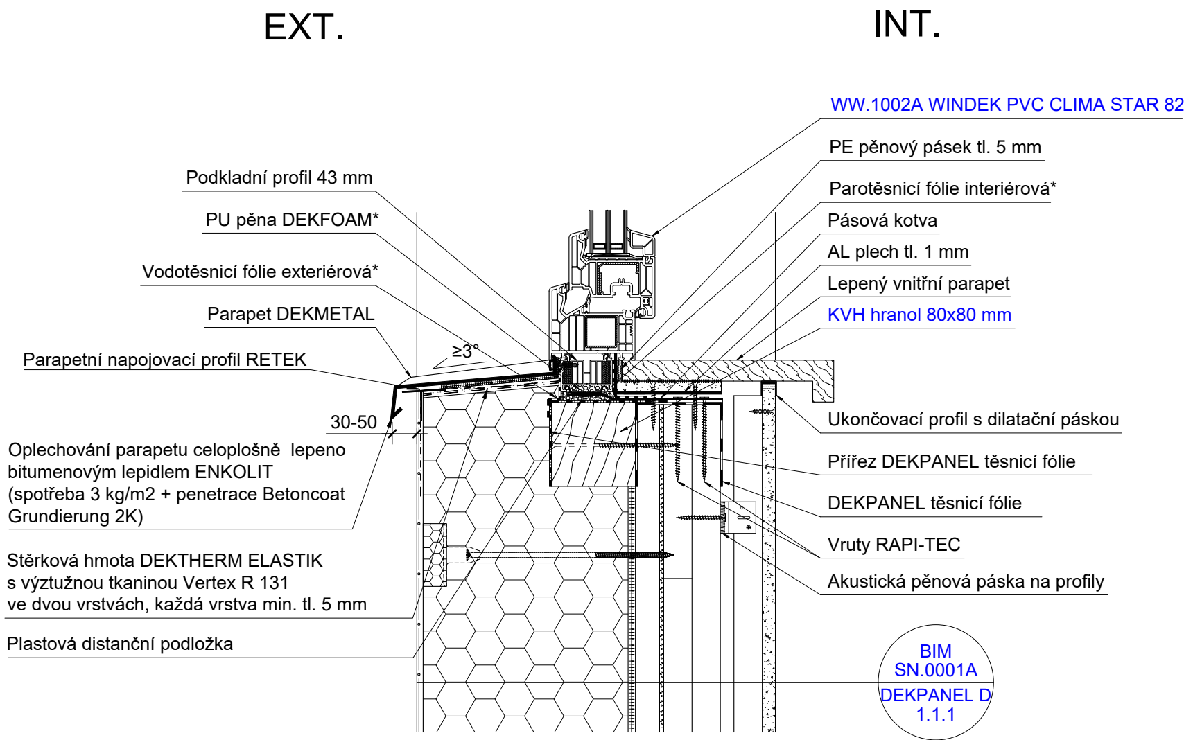
Řešení osazení okna do rámu z KVH hranolů
