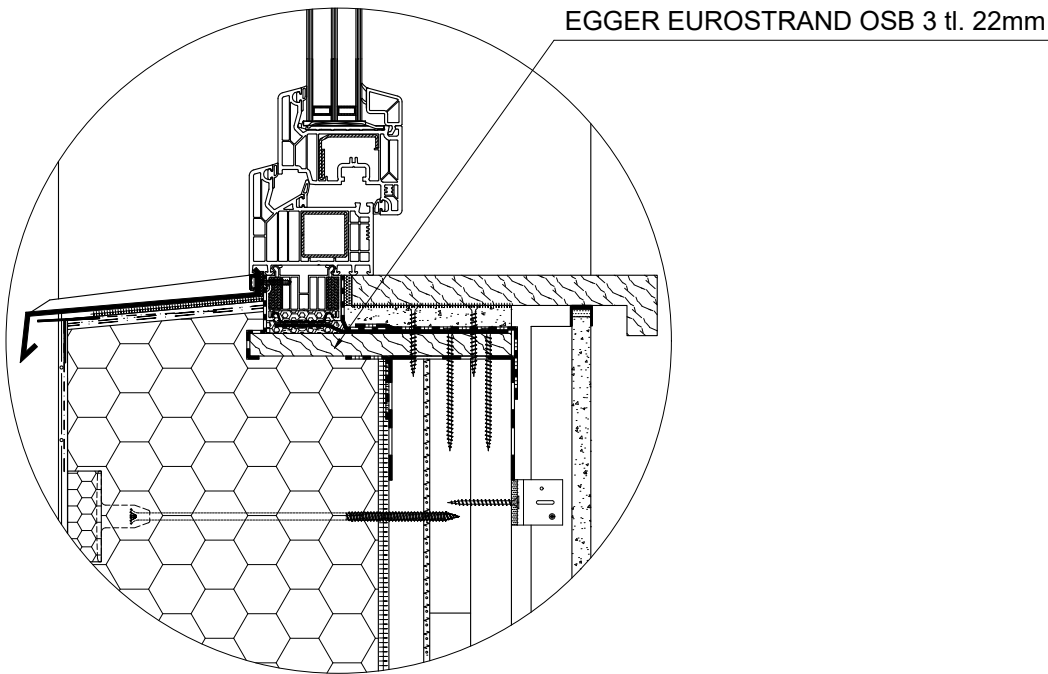
Řešení osazení okna do rámu z OSB desek
