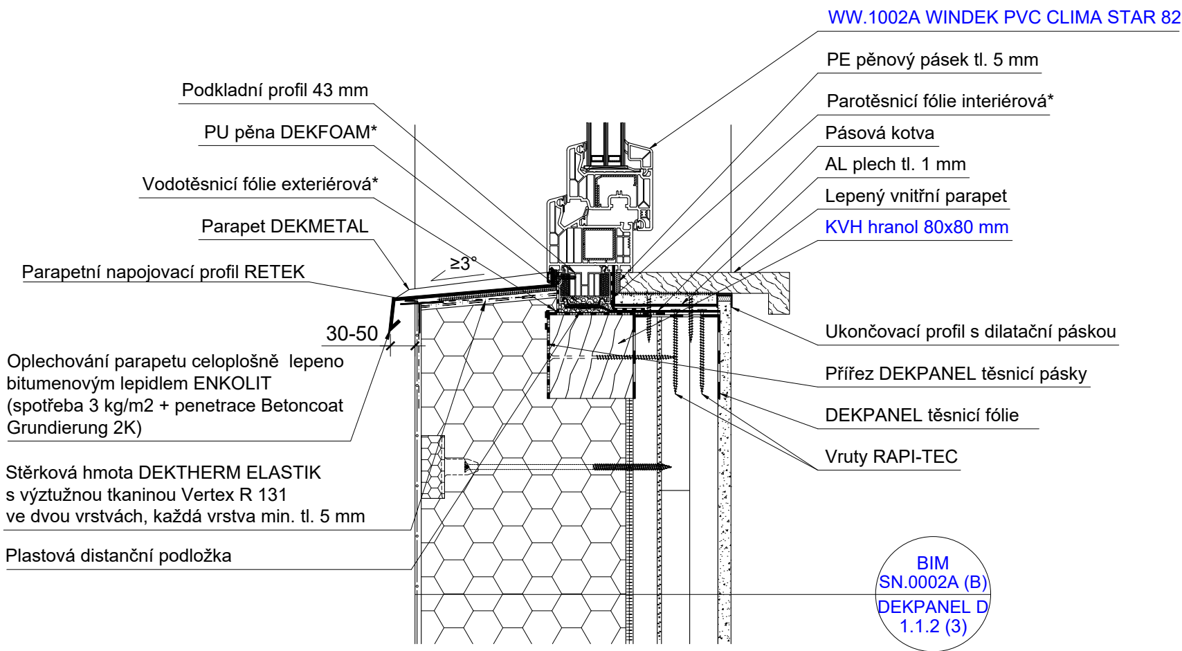
Řešení osazení okna do rámu z KVH hranolů
