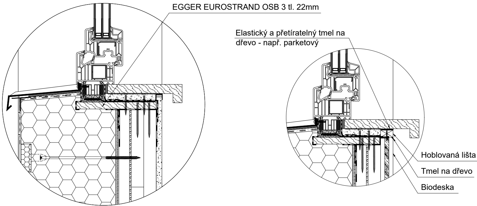
Řešení osazení okna do rámu z OSB desek
