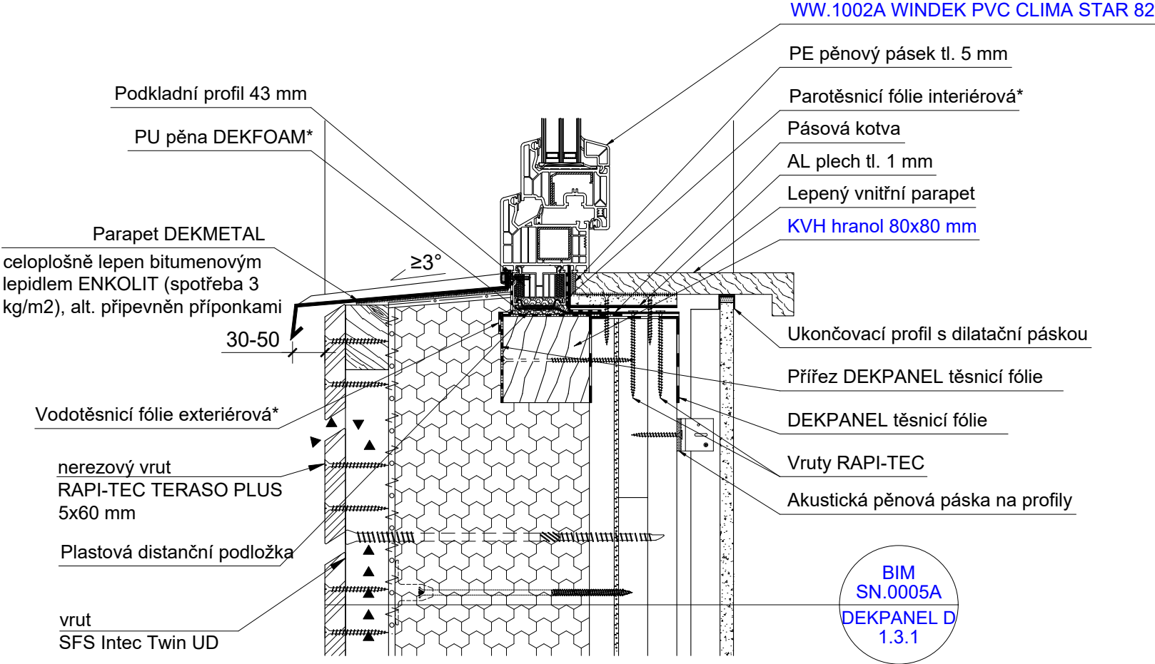
Řešení osazení okna do rámu z KVH hranolů
