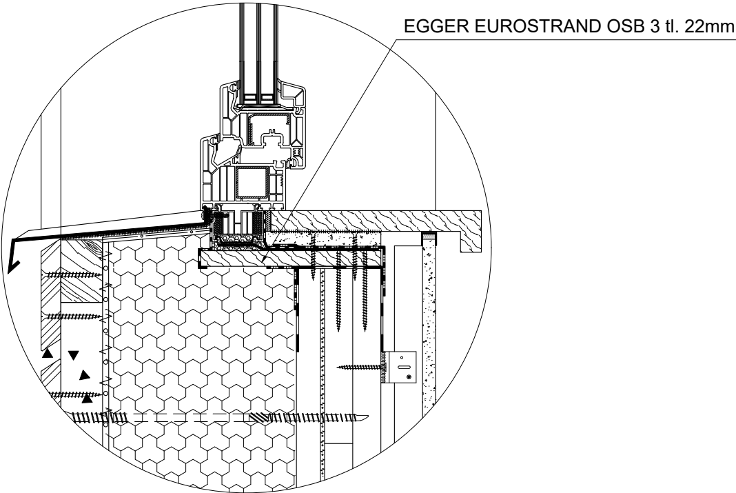
Řešení osazení okna do rámu z OSB desek
