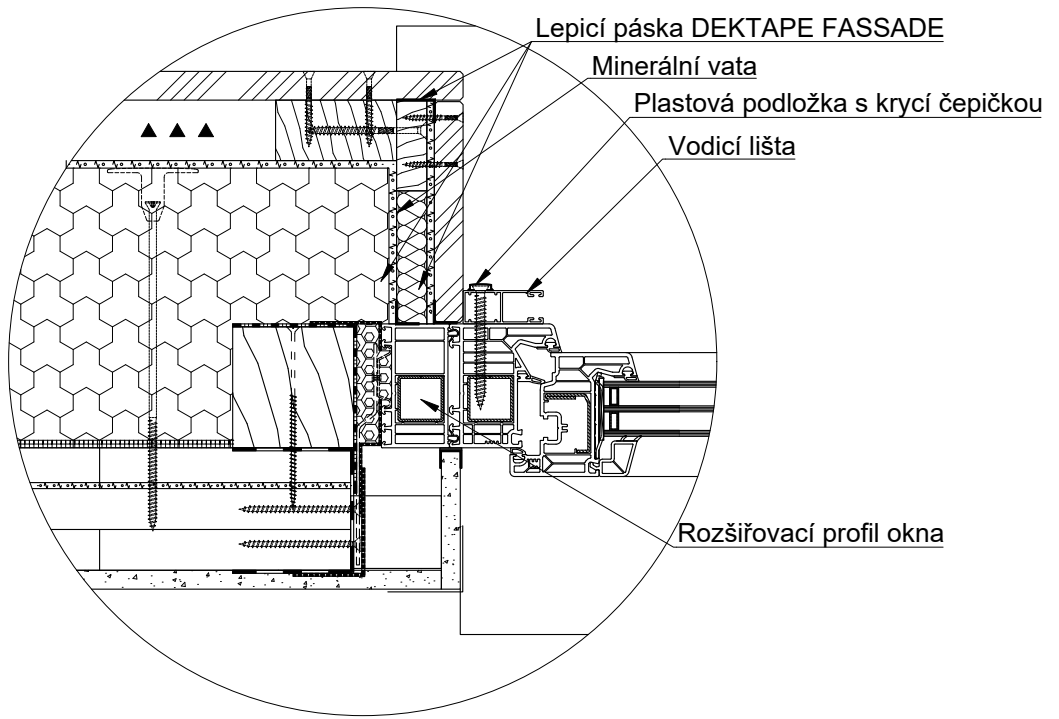
Řez ostěním s dřevěným obkladem a s příznanou vodící lištou
