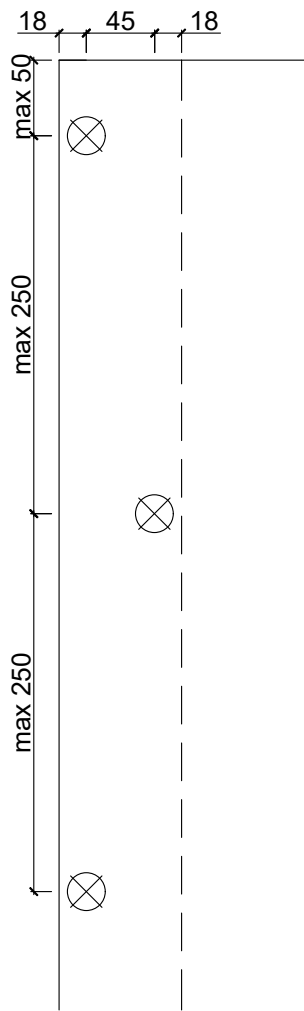
Spojení panelů vruty
