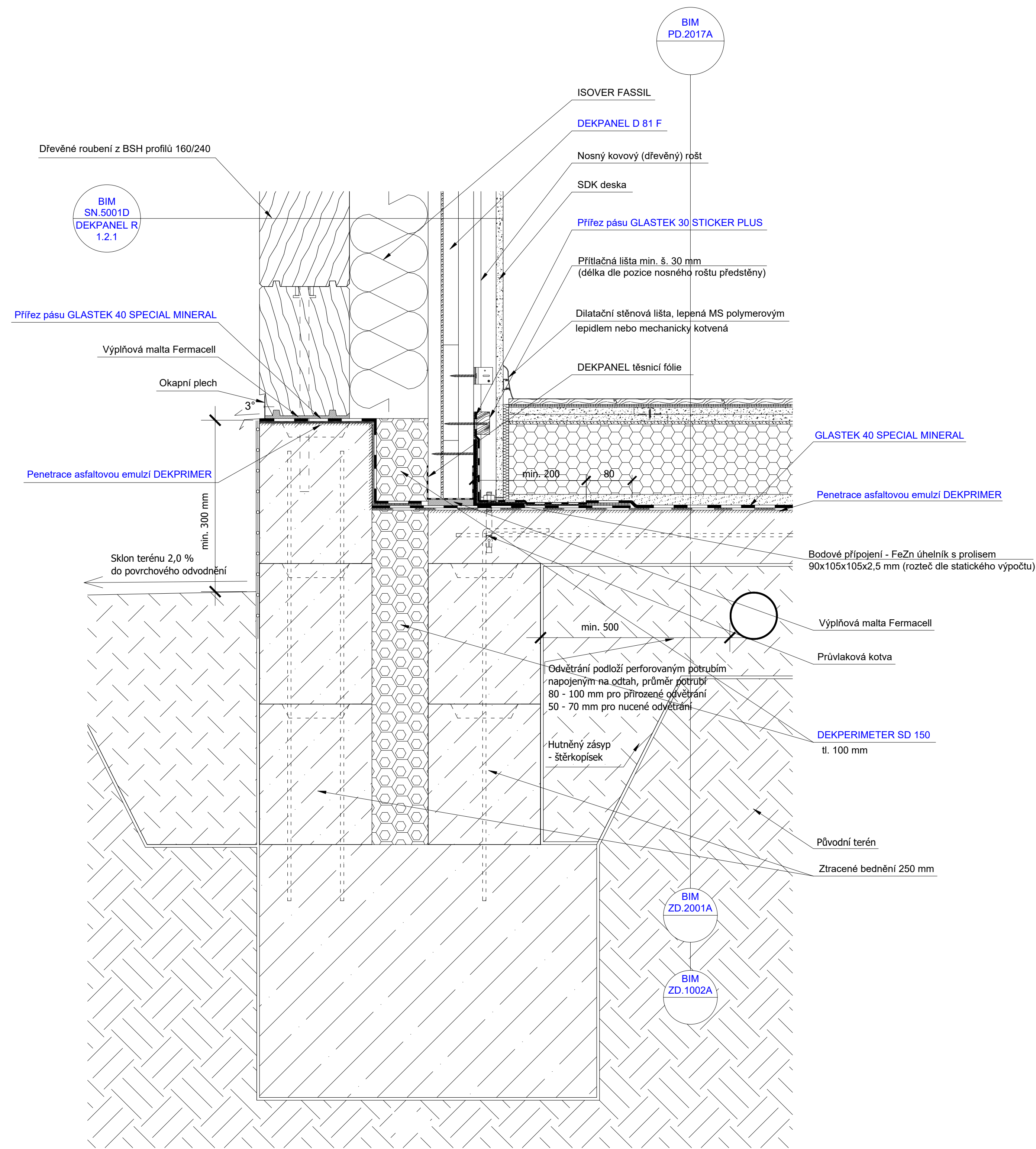
Řešení U.T. kolem objektu a soklové části viz detail ZD.2001A.
