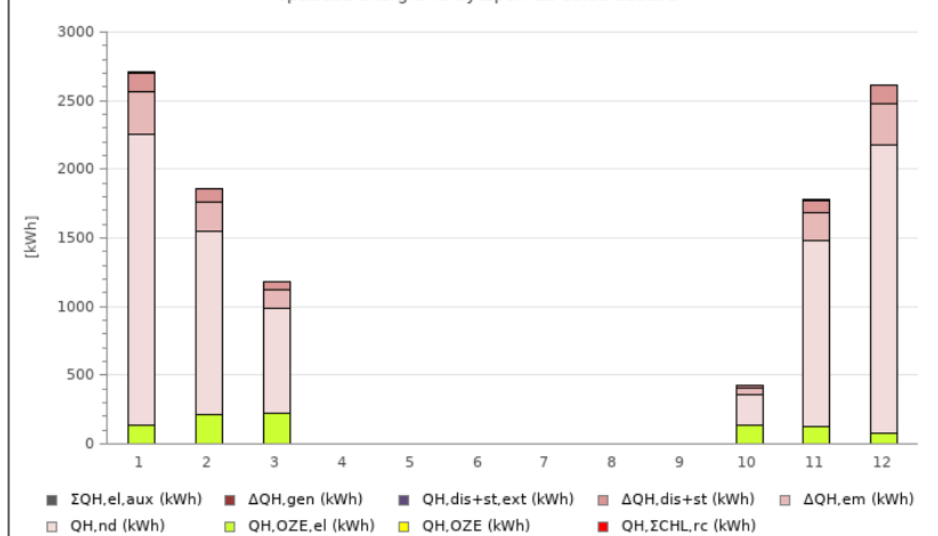
spotřeba energie na vytápění za celou budovu
