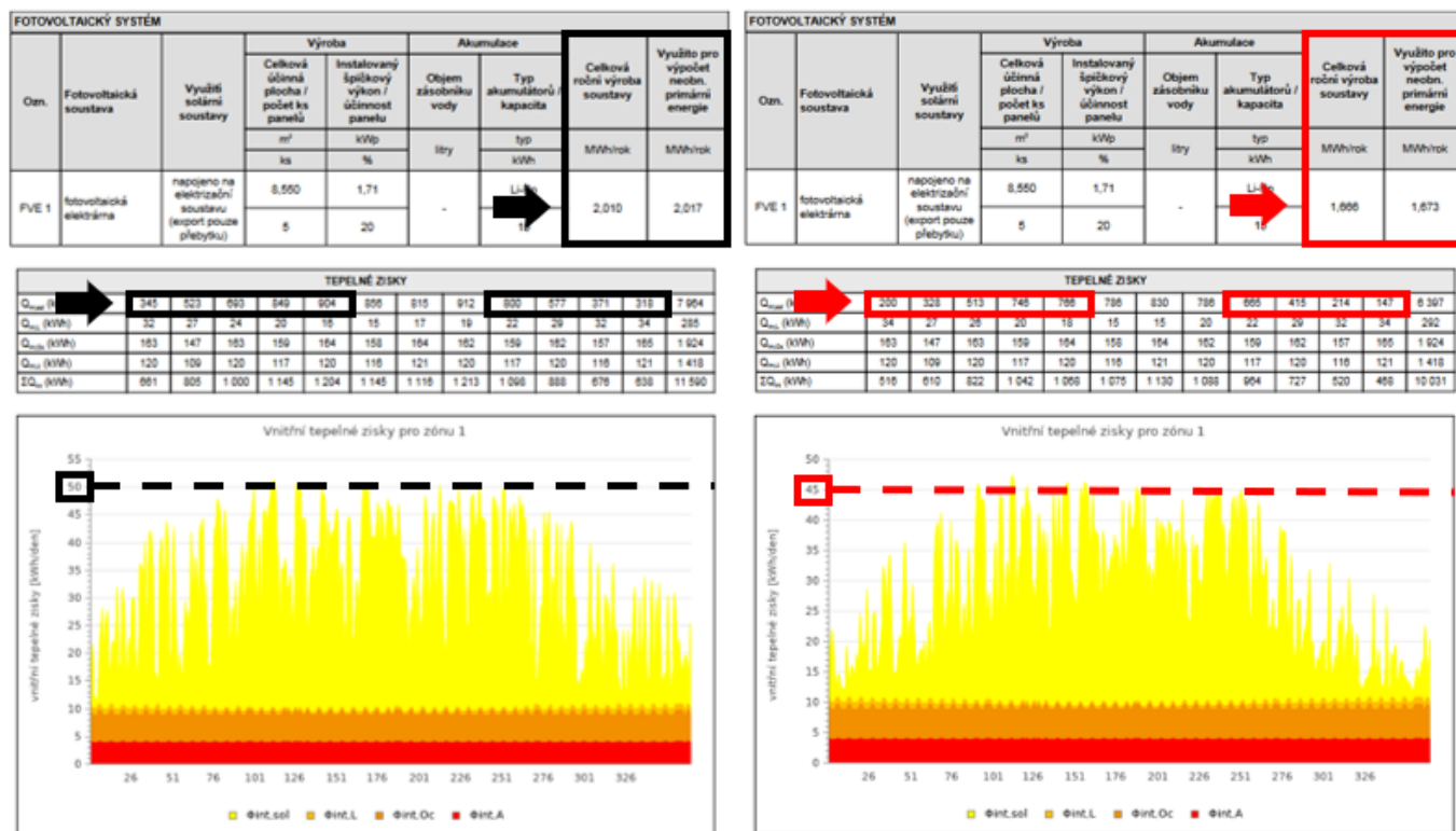
Obrázek 4 (vlevo): Produkce FVE a solární zisky vypočteny s klimadaty pro konkrétní lokalitu (Nemocnice Břeclav RKR 2009-2023).
